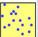
pure random
