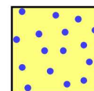
Poisson disk
